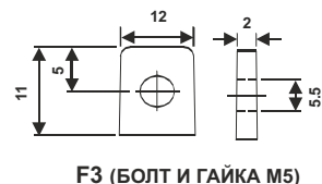
F3 (БОЛТ И ГАЙКА M5)
